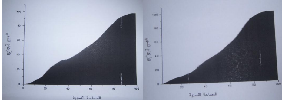
المنحنى الهيسومتري لحوض وادي بئر الواعر
