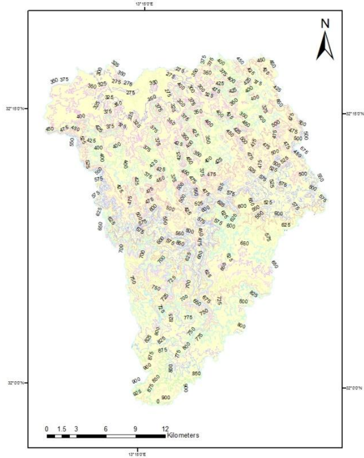
شكل (4) الخريطة الكنتورية لحوض وادي المجين
