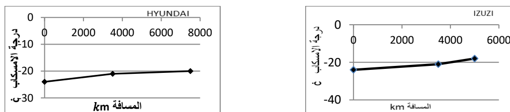
شكل 13. درجة الانسكاب للمحركين Pour point (مصفاة الزاوية)
