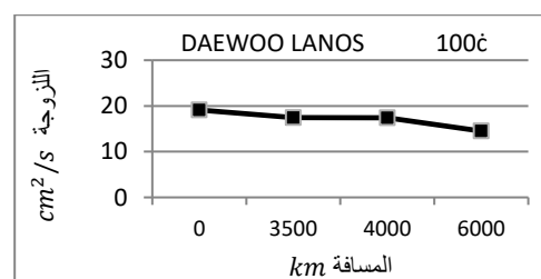
شكل 6. لزوجة الزيت SW50-10 عند درجات الحرارة 100°C (مصفاة الزاوية)
