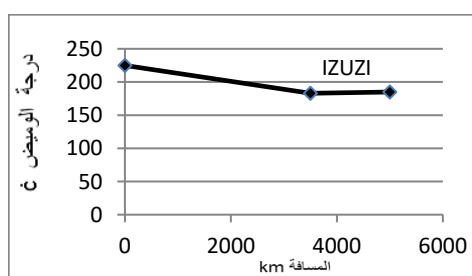
شكل 11. درجة الوميض للمحركين Flash point (مصفاة الزاوية)
