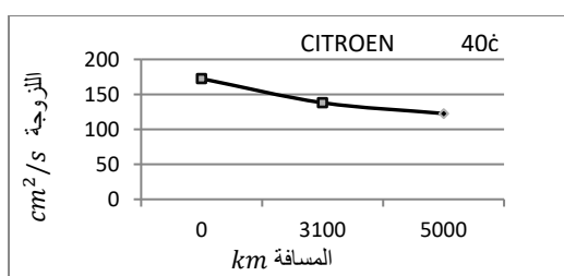
شكل 3. لزوجة الزيت SW50-10 عند درجات الحرارة 40^{\circ}\text{C} (مركز بحوث النفط)
