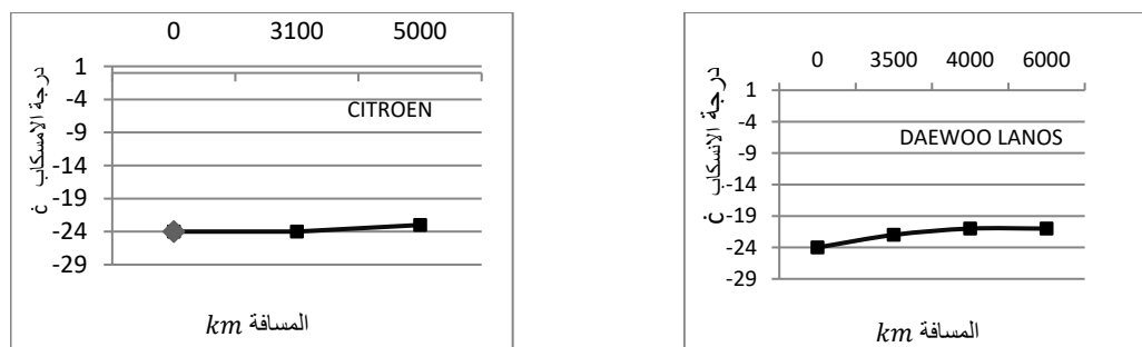
شكل 12. درجة الانسكاب للمحركين Pour point (مركز بحوث النفط)
