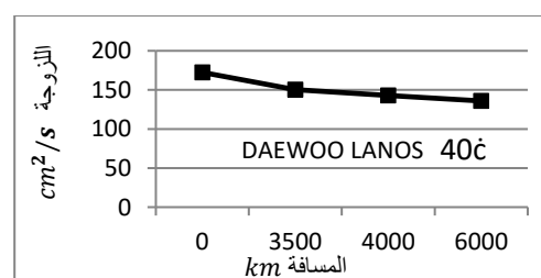
شكل 3. لزوجة الزيت SW50-10 عند درجات الحرارة 40^{\circ}\text{C} (مركز بحوث النفط)
